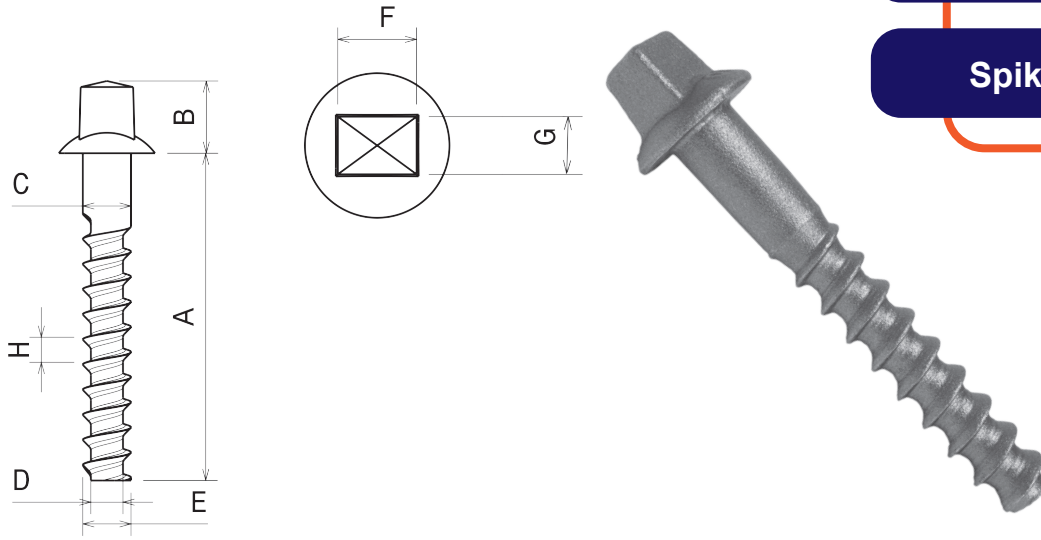
پیچ تراورس
